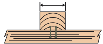
indirektes Auflager
